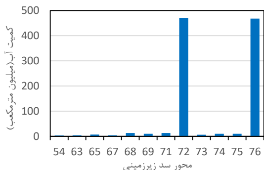
شکل ۷- مقایسه محورها بر اساس کمیت آب
