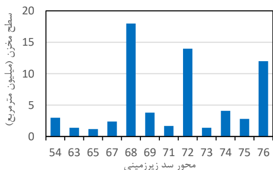
شکل ۵- مقایسه محورها بر اساس سطح مخزن
