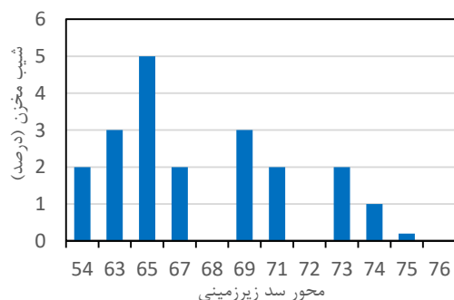
شکل ۴- مقایسه محورها بر اساس شیب مخزن
