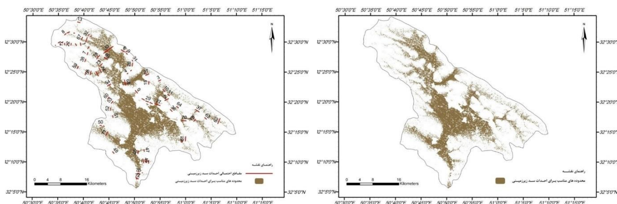
شکل ۱۸- تلفیق مقاطع احتمالی و محدوده‌های مناسب احداث سدهای زیرزمینی
