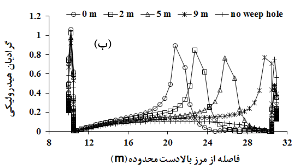
شکل ۴- تأثیر موقعیت سوراخ آب (مدل‌های شماره ۴ تا ۷): الف) توزیع زیر فشار، ب) توزیع گرادیان هیدرولیکی
