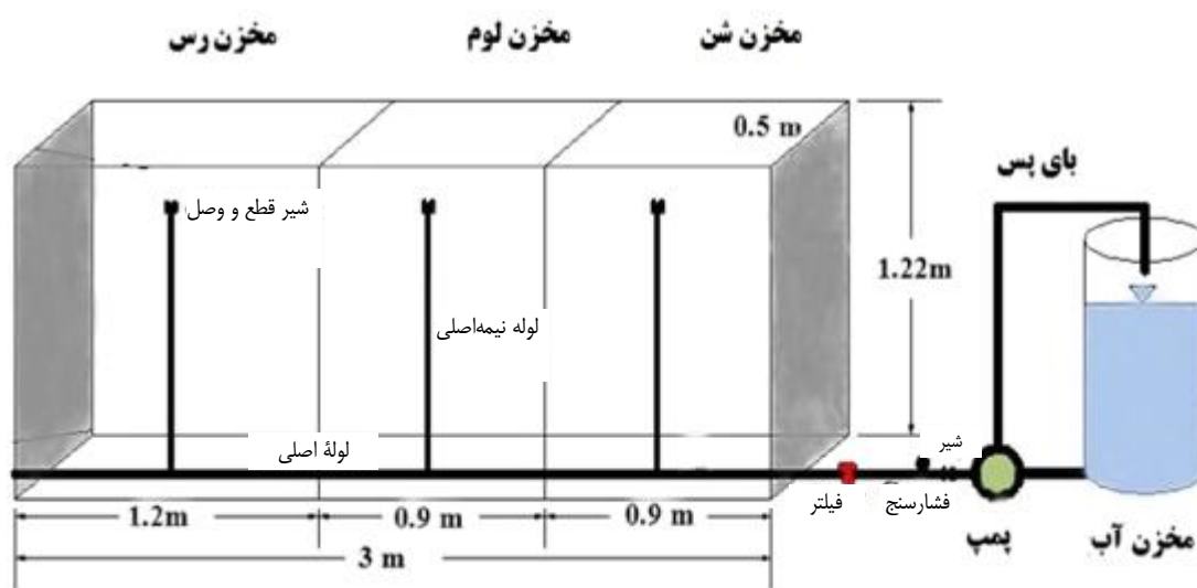
شکل ۱- لایسیمتر آزمایشگاهی و اتصالاتی مربوط به آزمایش
