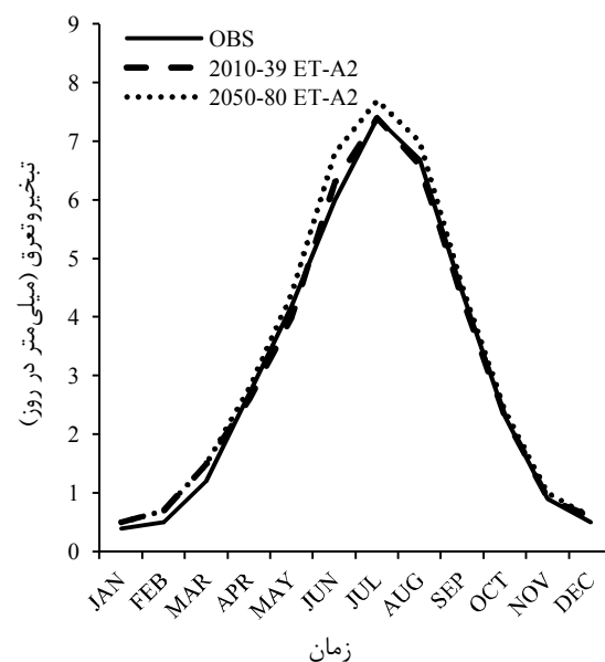
شکل ۴- تغییرات تبخیر و تعرق در سه دوره مطالعاتی (۱۹۷۰-۲۰۰۰) (OBS)، (۲۰۱۰-۳۹) و (۲۰۵۰-۸۰)
