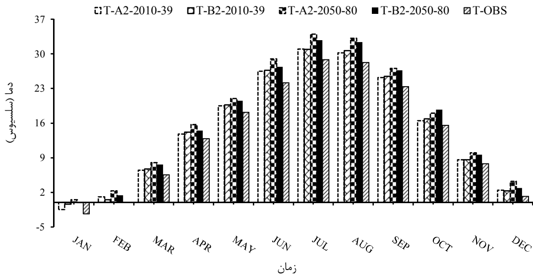
شکل ۲- تغییرات دما در سه دوره مطالعاتی (OBS) ۱۹۷۰-۲۰۰۰، ۲۰۱۰-۳۹ و ۲۰۵۰-۸۰
