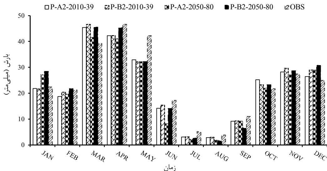
شکل ۳- تغییرات بارش در سه دوره مطالعاتی (OBS) ۱۹۷۰-۲۰۰۰، ۲۰۱۰-۳۹ و ۲۰۵۰-۸۰
