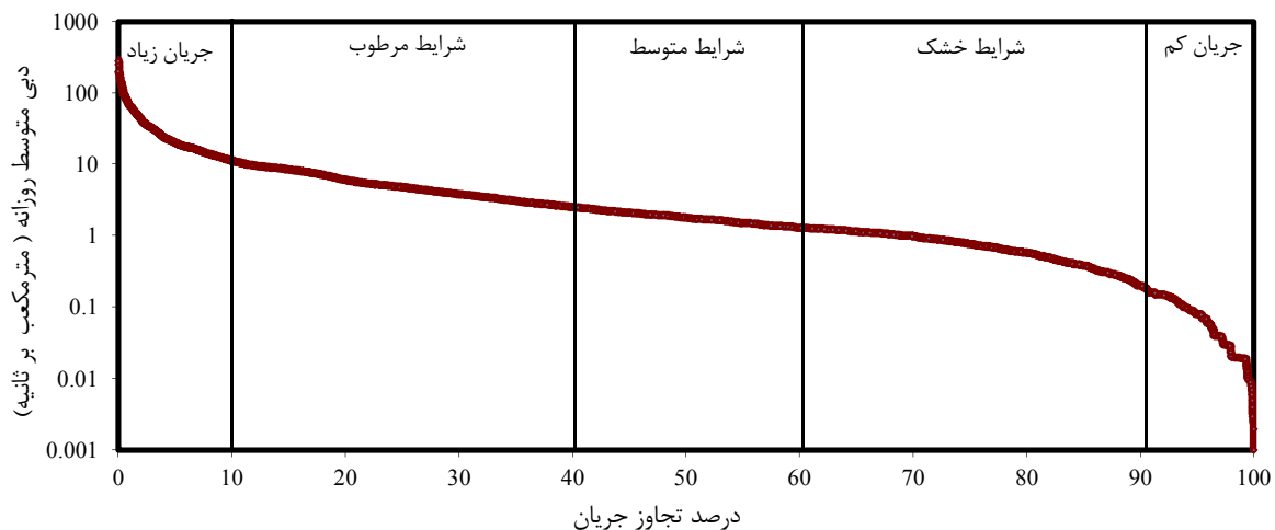
شکل ۲- نمونه منحنی تداوم جریان برای جریان ۳۰ ساله (سازمان حفاظت محیط‌زیست، ۲۰۰۷)
