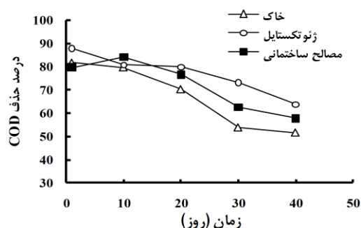
شکل ۳- تغییرات درصد حذف کل BOD 5 نسبت به زمان در ستون‌ها
