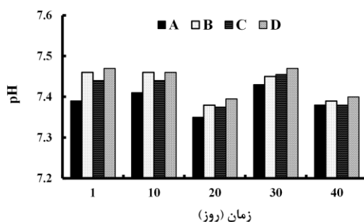
شکل ۵- مقادیر میانگین pH پساب ورودی (A) و خروجی از انتهای ستون بدون پوشش (B)، ستون دارای پوشش ژئوتکستایل (C) و ستون با پوشش مصالح (D) در طول دوره آزمایش
