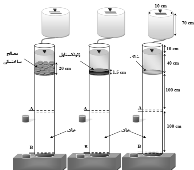
شکل ۱- شمای کلی مدل فیزیکی ساخته شده در اجرای عملیات تغذیه مصنوعی با فاضلاب
