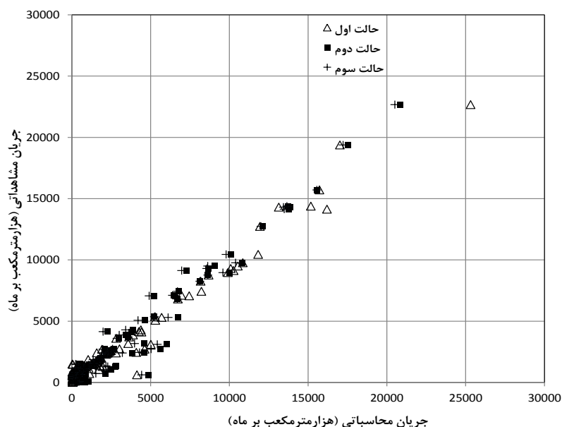
شکل ۸- نمودار پراکنش داده‌های جریان سطحی
