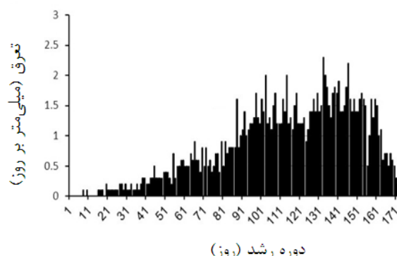
شکل ۱- مقادیر تبخیر از سطح خاک (سمت چپ) و تعرق از گیاه (سمت راست) در مزرعه A (چهار هکتاری) با استفاده از مدل AquaCrop
