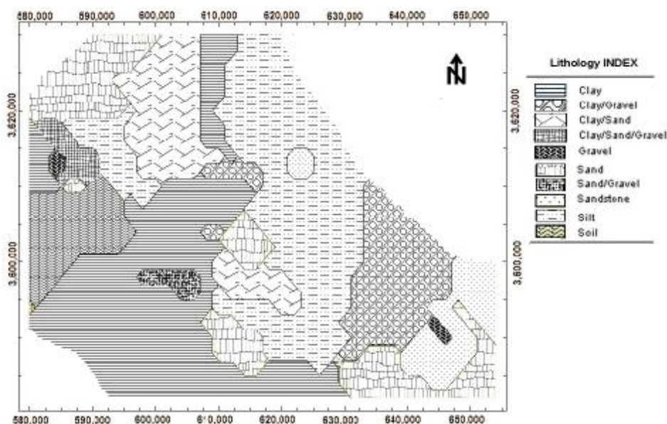
شکل 4- پلان زمین‌شناسی دشت ورزنه، بر اساس داده‌های لاگ لیتولوژی برای عمق 1480
