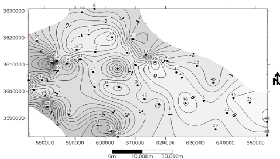
شکل 6- نقشه هم‌افت آب زیرزمینی بین سال 1376 و 1386 در دشت ورزنه* * شماره پیژومترها داخل مربع نوشته شده است.
