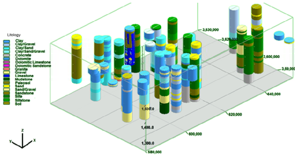
شکل 3- لاگ‌های حفاری چاه‌های دشت ورزنه
