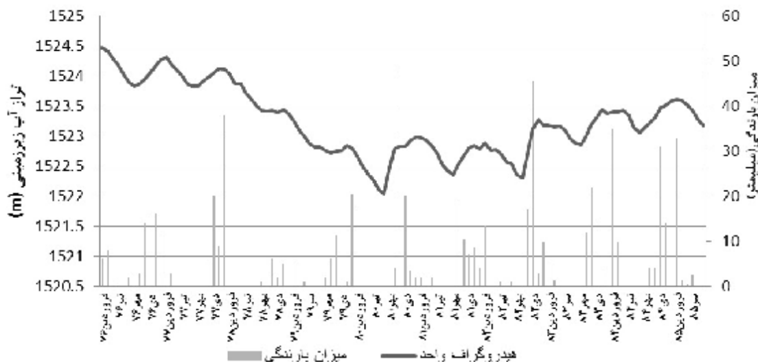
شکل 5- مقایسه هیدروگراف میانگین و میانگین بارندگی دشت ورزنه
