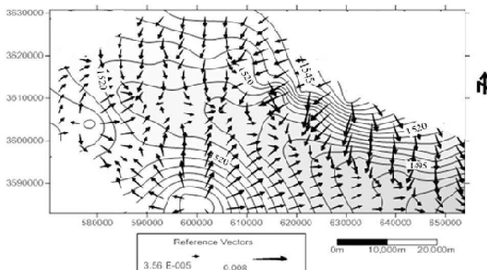
شکل 11- جهت جریان آب در دشت ورزنه (خرداد 1387)
