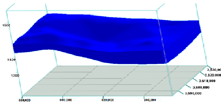
شکل ۹- مدل لایه آبدار تحت فشار در دشت ورزنه
