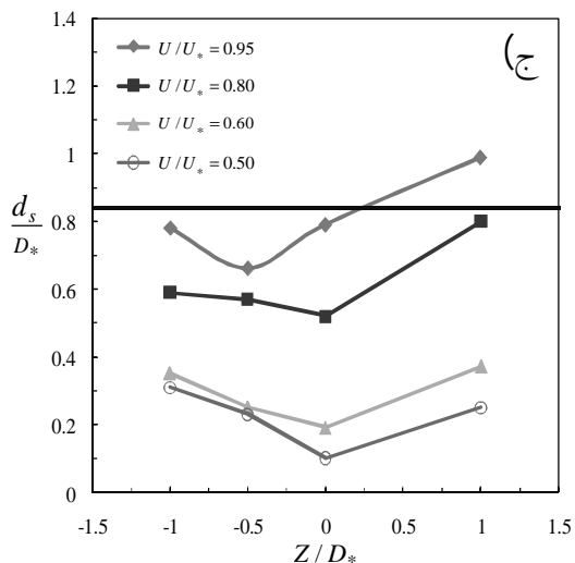
شکل 6- مقایسه تغییرات عمق نهایی آبشستگی برای شرایط مختلف هیدرولیکی و ترازهای کارگذاری فونداسیون، (الف) عمق نسبی y/D_* = 1 ، (ب) عمق نسبی y/D_* = 2 و (ج) y/D_* = 3
