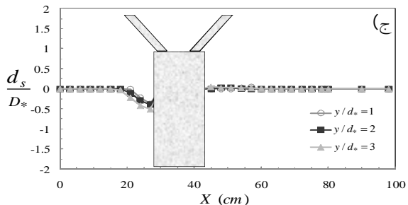
شکل 5- نیمرخ نهایی آبشستگی برای شرایط هیدرولیکی مختلف و رقوم کارگذاری Z/D_* = 1 (الف) U/U_c = 0.95 ، (ب) U/U_c = 0.8 ، و (ج) U/U_c = 0.6
