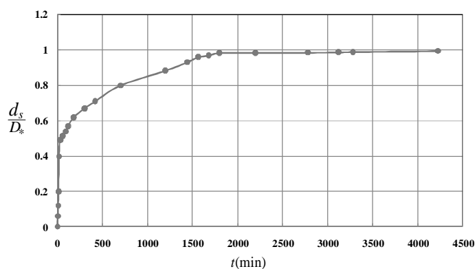
شکل 2- توسعه زمانی آبشستگی برای U/U_c = 0.95 , y/D_* = 1 , و Z/D_* = 0
