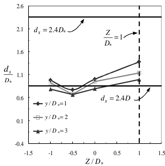
شکل 8- تغییرات حداکثر عمق آب‌شستگی برای سرعت نسبی U/U_c = 0.95 و عمق‌های نسبی مختلف
