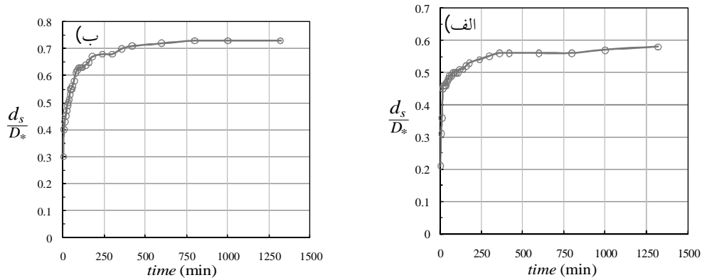
شکل 7- توسعه زمانی آب‌شستگی در مقابل پایه پل در وضعیت رقوم کارگذاری فونداسیون برابر Z/D_* = -0.5 ، الف) U/U_c = 0.95 و y/D_* = 1 و ب) U/U_c = 0.8 و y/D_* = 3
