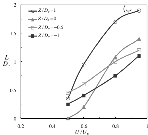
شکل 9- تغییرات حداکثر طول آب‌شستگی مقابل پایه برای شرایط مختلف هیدرولیکی و رقوم کارگذاری فونداسیون، الف) عمق نسبی جریان y/D_* = 1 و ب) عمق نسبی جریان y/D_* = 3
