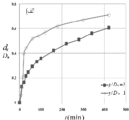
شکل 3- تغییرات زمانی عمق آبشستگی برای شرایط هیدرولیکی مختلف در تراز کارگذاری Z/D_* = 0
