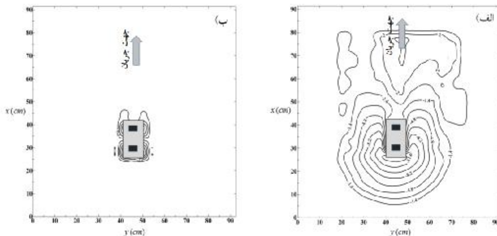
شکل 4- مقایسه تغییرات خطوط تراز تغییرات بستر در مجاورت پایه پل در رقوم کارگذاری Z/D_* = 1
