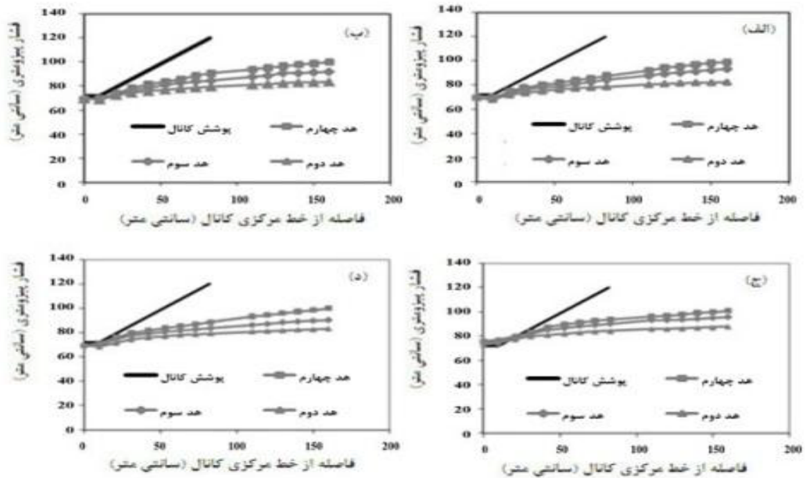
شکل ۶- نیمرخ نشت بازای زهکش ژئونت به ضخامت ۲۴ میلی‌متر؛ در شرایط اعمال وزن: الف) GT300-1؛ ب) GT250؛ ج) GT300-2؛ د) GT150
