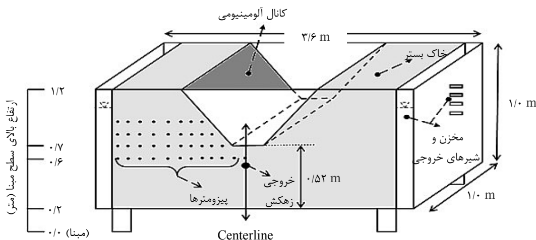
شکل ۱- نمای شماتیکی از مدل فیزیکی و اجزای آن
