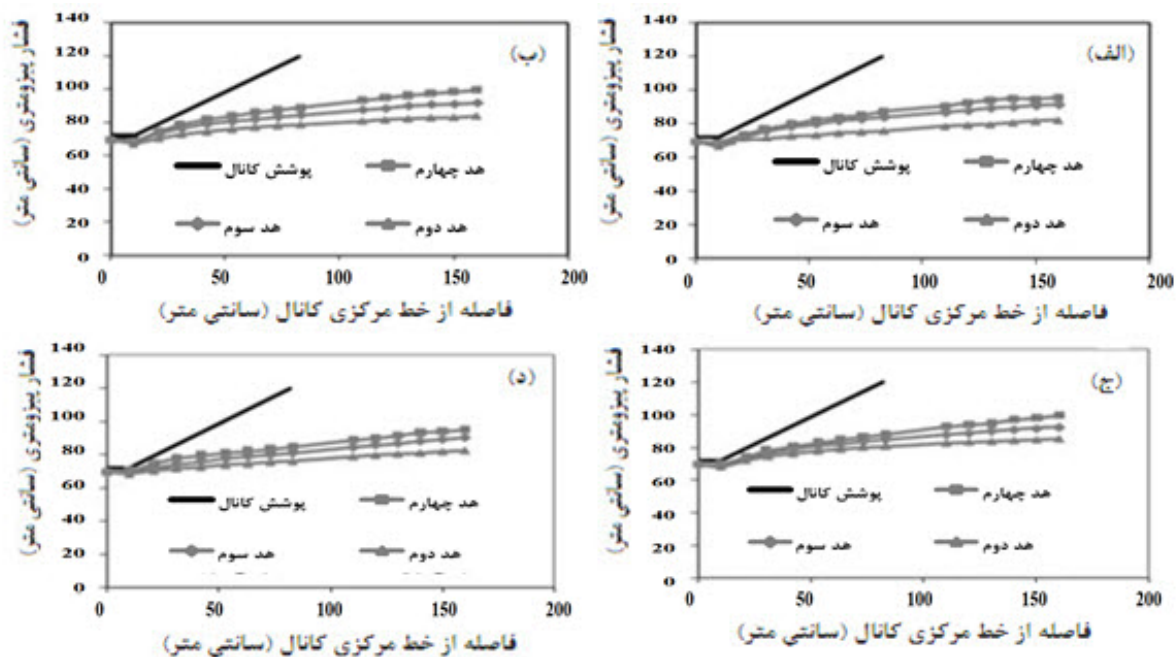
شکل ۴- نیمرخ نشت بازای زهکش ژئونت به ضخامت ۲۴ میلی‌متر؛ بدون اعمال وزن: الف) GT 300-1؛ ب) GT 250؛ ج) GT 300- د) GT 150
