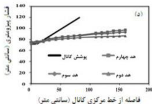
شکل ۳- نیمرخ نشت بازای زهکش ژئونت به ضخامت ۱۲ میلی‌متر؛ بدون اعمال وزن: الف) GT 300-1 (ب) GT 250 (ج) GT 300-2 (د) GT 150
