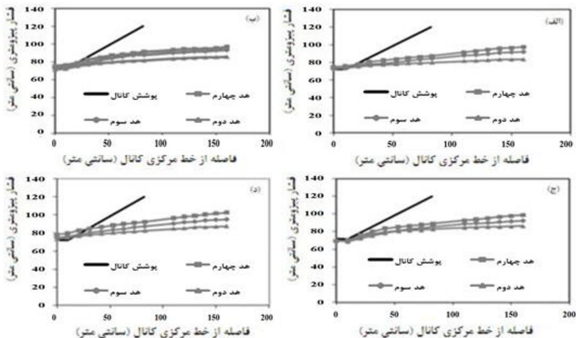
شکل ۵- نیمرخ نشت بازای زهکش ژئونت به ضخامت ۱۲ میلی‌متر؛ در شرایط اعمال وزن: الف) GT 300-1؛ ب) GT 250؛ ج) GT 300- د) GT 150
