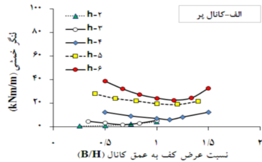
شکل ۵- تغییرات لنگر خمشی وارده بر پوشش بتنی به ازای ابعاد مختلف کانال دوزنقه‌ای با شیب ۱:۲
