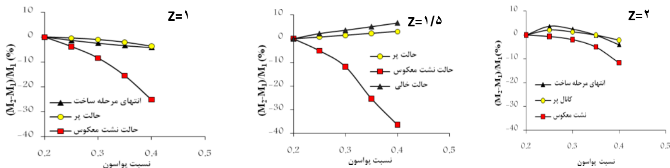
شکل ۷- تغییرات لنگر وارده بر دیواره جانبی کانال‌های آبیاری در مقادیر مختلف نسبت بواسون
