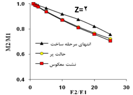
شکل ۶- تغییرات لنگر وارده بر دیواره جانبی کانال‌های آبیاری در مقادیر مختلف مدول الاستیسیته خاک در شیب‌های جانبی مختلف
