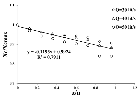
شکل ۹- تغییرات محل تشکیل عمق بحرانی با افزایش ارتفاع رسوبات در پشت سرریز
