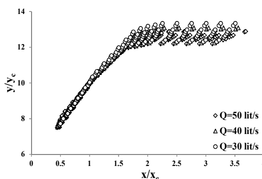
شکل ۷- پروفیل بدون بعد بعد سطح آب روی سرریز
