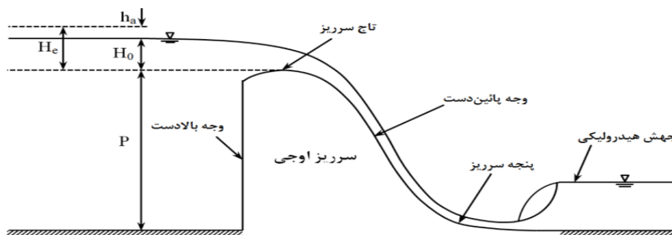
شکل ۱- نمایی از یک سرریز اوجی و قسمت‌های مختلف آن (شوشتری، ۱۳۸۷)
