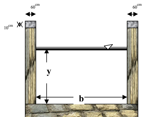
شکل ۲- مقطع عمومی جریان در کانال‌های مورد بررسی
