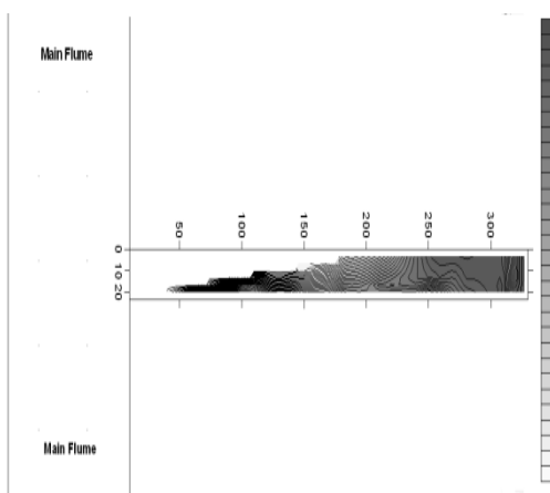
شکل ۱۰- توپوگرافی بستر کانال آبگیر (نسبت دبی ۰/۶)
