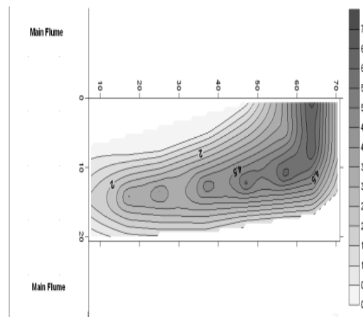
شکل ۹- توپوگرافی بستر کانال آبگیر
