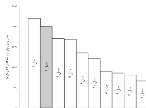
شکل ۷- مقایسه بین نتایج به دست آمده از وزن رسوبات وارد شده به آبگیر (نسبت دبی ۰/۲)
