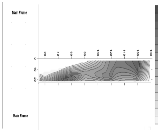
شکل ۸- توپوگرافی بستر کانال آبگیر
