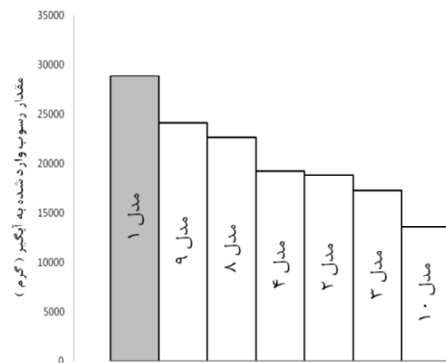
شکل ۵- مقایسه بین نتایج به دست آمده از وزن رسوبات وارد شده به آبگیر (نسبت دبی ۰/۶)
