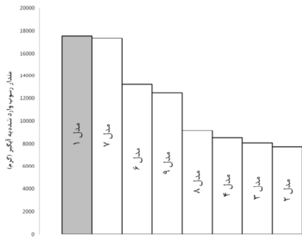
شکل ۶- مقایسه بین نتایج به دست آمده از وزن رسوبات وارد شده به آبگیر (نسبت دبی ۰/۴)
