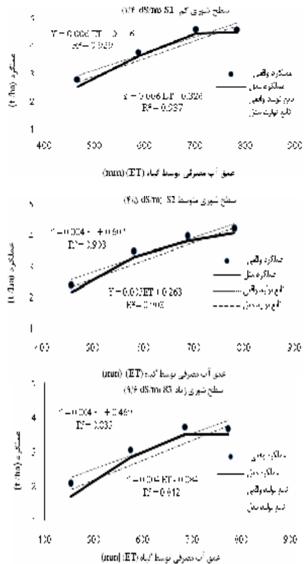
شکل ۳- نمودار توابع تولید گندم نسبت به عمق آب مصرفی برای مدل و شرایط مزرعه در سطوح شوری مختلف
