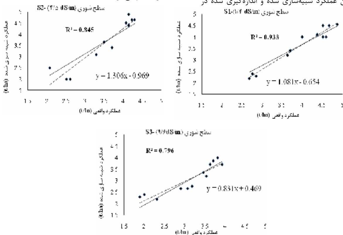
شکل ۷ - نتایج صحت‌یابی مدل SWAP برای شبیه‌سازی عملکرد در سطوح شوری مختلف
