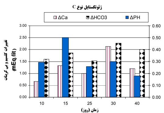
شکل ۸- تغییرات پارامترهای شیمیایی برای ژئوتکستایل نوع C
