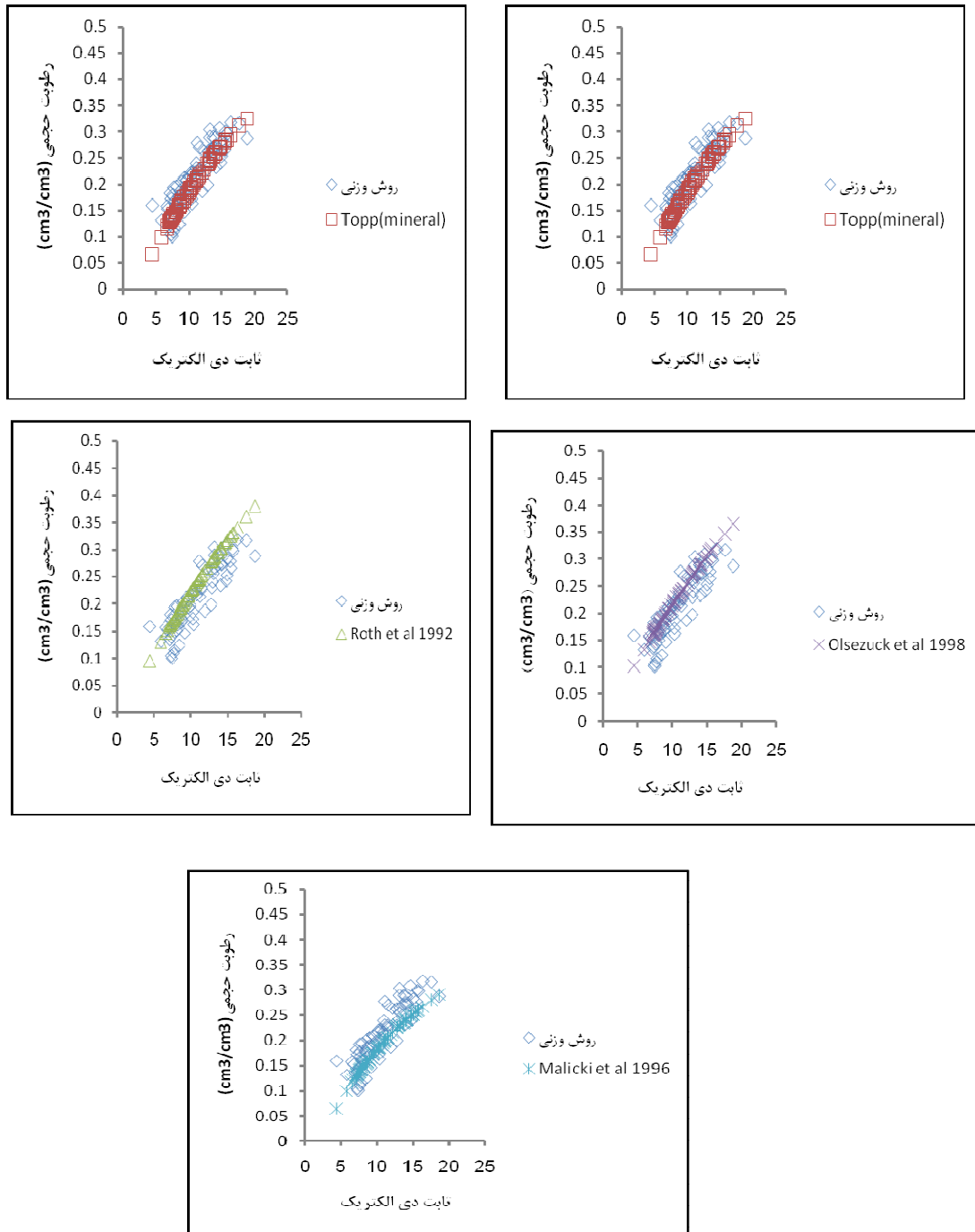
شکل (۱) - نمودار رطوبتی به دست آمده به روش وزنی و مدل‌ها به صورت تابعی از ثابت دی‌الکتريک در بافت سبک. اشکال a, b, c, d, e به ترتیب مقایسه روش وزنی با مدل‌های تاپ، راس، اولسزوک، مالیکی و ترکیبی است
