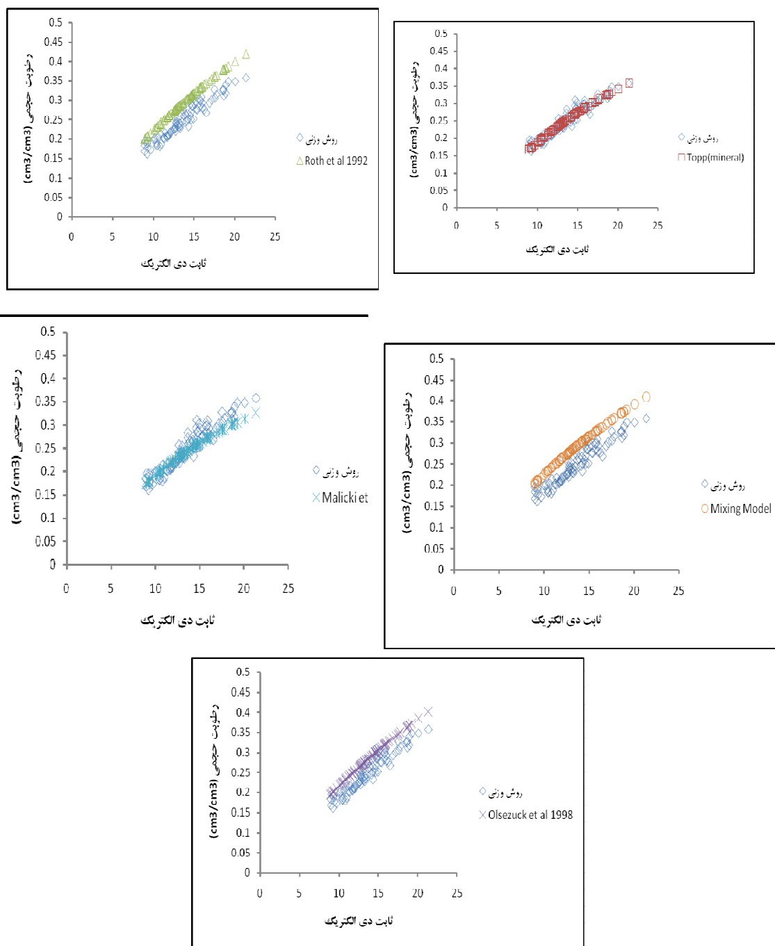
شکل ۲- نمودار رطوبتی به دست آمده به روش وزنی و مدل‌ها به صورت تابعی از ثابت دی الکتریک در بافت متوسط، اشکال a, b, c, d, e به ترتیب مقایسه روش وزنی با مدل‌های تاپ، راس، اولسزوک، مالیکی و ترکیبی است
