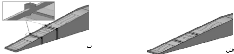
شکل ۴- سرریز مدل‌سازی شده (الف) با هواده‌ی رمپ، (ب) با هواده‌ی ترکیب رمپ و داکت هواده
