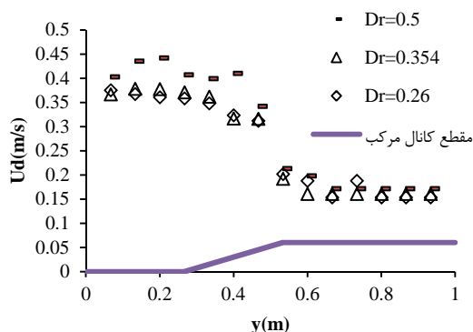
شکل ۳- توزیع سرعت متوسط عمقی با وجود پوشش گیاهی در شیب ۰/۰۰۱۵، در ۶/۵ متری از ابتدای فلوام الف) تراکم (۱/۱۶/۶) در تراکم ۱۶۶۷ ب)
