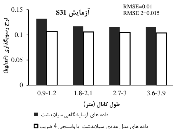
شکل ۵- مقایسه نرخ رسوب‌گذاری آزمایشگاهی با نرخ رسوب‌گذاری حاصل از مدل عددی
