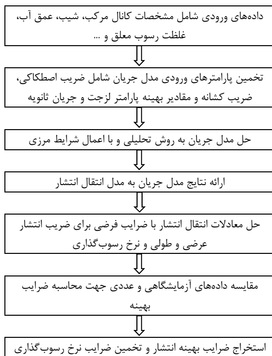
شکل ۲- شمای کلی مدل عددی
