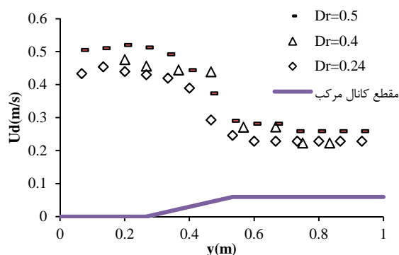
شکل ۳- توزیع سرعت متوسط عمقی با وجود پوشش گیاهی در شیب ۰/۰۰۱۵، در ۶/۵ متری از ابتدای فلوام الف) تراکم (۱/۱۶/۶) در تراکم ۱۶۶۷ ب)
