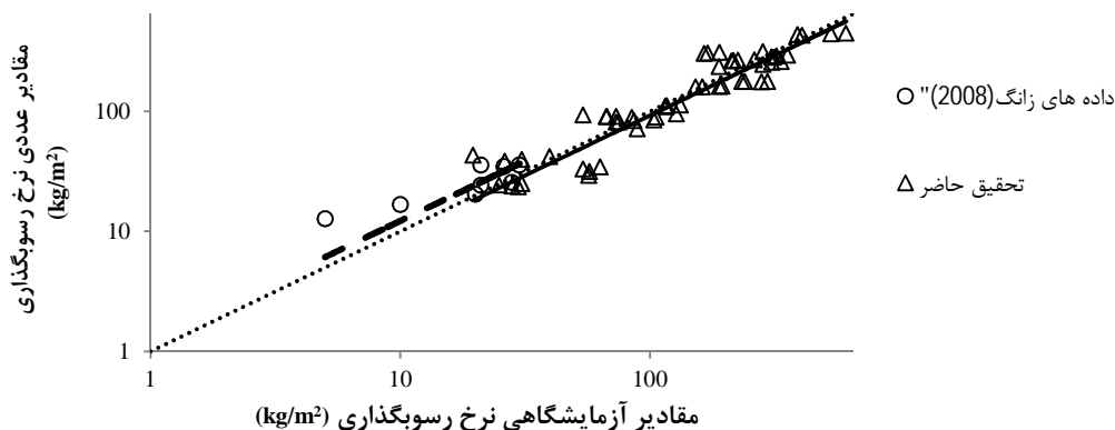
شکل ۶- مقایسه نتایج مدل عددی و داده‌های آزمایشگاهی
