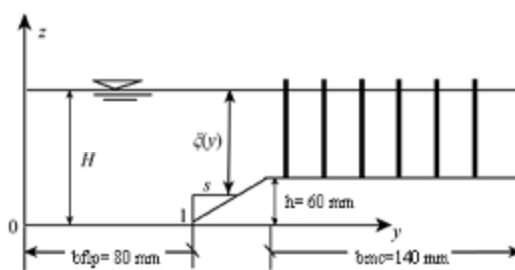
شکل ۱- مقطع عرضی کانال مرکب
