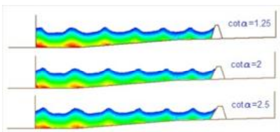
شکل ۹- نمایش بالاروی موج در حالت شیب‌های مختلف بدنه موج‌شکن (۲/۵ و ۲ و ۱/۲۵) (روش SPH)
