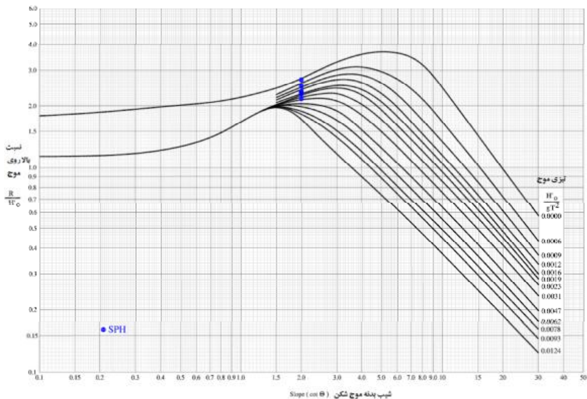
شکل ۱۳- مقایسه میزان بالاروی با توجه به رابطه تیزی موج و شیب بدنه موج شکن با استفاده از روش هیدرودینامیک ذرات هموار در مدل دوم و نتایج آزمایشگاهی ارائه شده توسط اداره مهندسی ارتش آمریکا (ارتش آمریکا، ۱۹۸۴)
