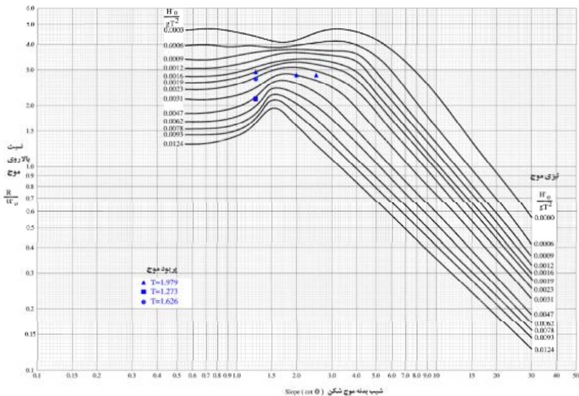
شکل ۶- مقایسه میزان بالاروی بر حسب زمان تناوب، تیزی و شیب پدنه موج شکن با استفاده از روش هیدرودینامیک ذرات هموار و نتایج آزمایشگاهی ارائه شده (خط ممتد) توسط اداره مهندسی ارتش آمریکا (ارتش آمریکا، ۱۹۸۴)
