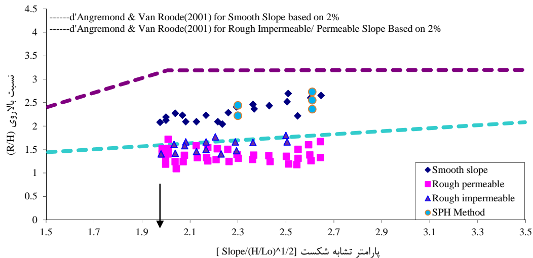
شکل ۱۲- مقایسه میزان بالاروی موج بر حسب پارامتر تشابه شکست برای مدل‌های موج‌شکن هموار (صلب) بر اساس دو روش آزمایشگاهی و SPH (شانکار و جایاراتنه، ۲۰۰۳)
