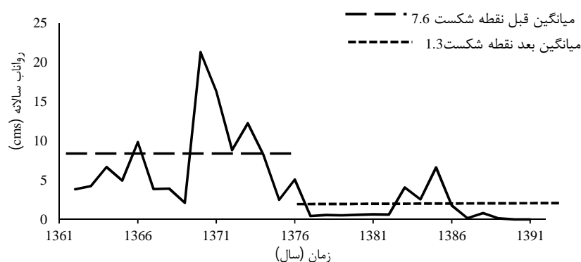
شکل ۳- تغییر در سری زمانی رواناب ایستگاه وسج
