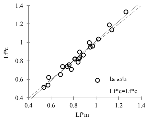
شکل ۴- مقایسه مقادیر محاسبه شده با مقادیر اندازه‌گیری شده آن‌ها
