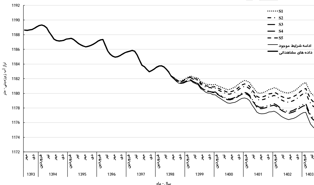
شکل ۱۲- هیدروگراف آبخوان در اعمال سیاست‌های تعادل بخشی تحت سناریوی انتشار RCP8.5 (S 1 تا S 5 ) به ترتیب سناریوهای مدیریتی بهره‌برداری از آبخوان هشتگرد با هدف بهبود تراز آب زیرزمینی و احیا و تعادل بخشی آن است.
