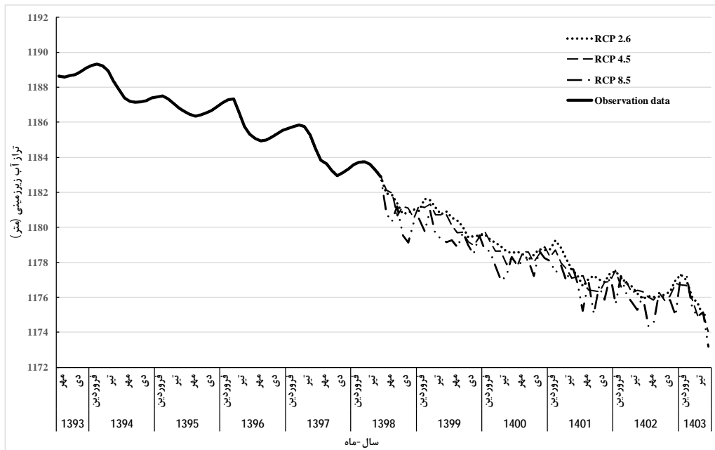
ج- GFDL-CM3
