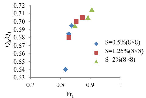
شکل ۷- رابطه دبی نسبی عبوری رأس در مقابل عدد فرود دسیمتریک مقطع اول
