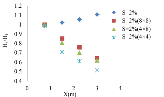
شکل ۵- تغییرات ارتفاع رأس جریان غلیظ نمکی برای سیال غلیظ ۱۰ گرم در لیتر در سه شیب ۰/۵، ۱/۲۵ و ۲ درصد
