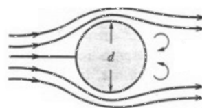
شکل ۳- خطوط جریان اطراف مانع استوانه‌ای شکل
