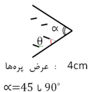
شکل ۴- حالات قرارگیری پره‌های هادی در آزمایش‌های گروه ۲
