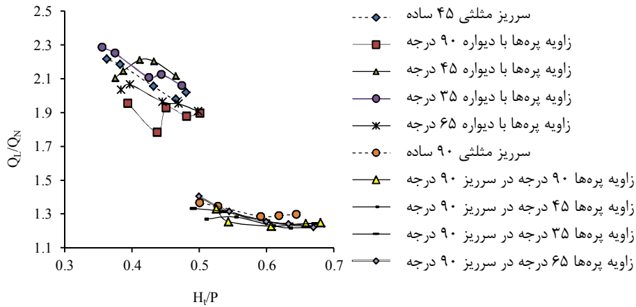
شکل ۱۳- مقایسه تغییرات بازده سرریز (Q L /Q N ) نسبت به H t /P در آزمایش‌های گروه ۲ در دو سرریز با زاویه وجه ۹۰ و ۴۵ درجه
