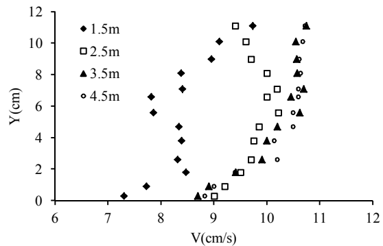
شکل ۷- نیمرخ‌های سرعت برداشت شده در فواصل ۲/۵، ۱/۵، ۳/۵ و ۴/۵ متری از ابتدا در محور مرکزی
